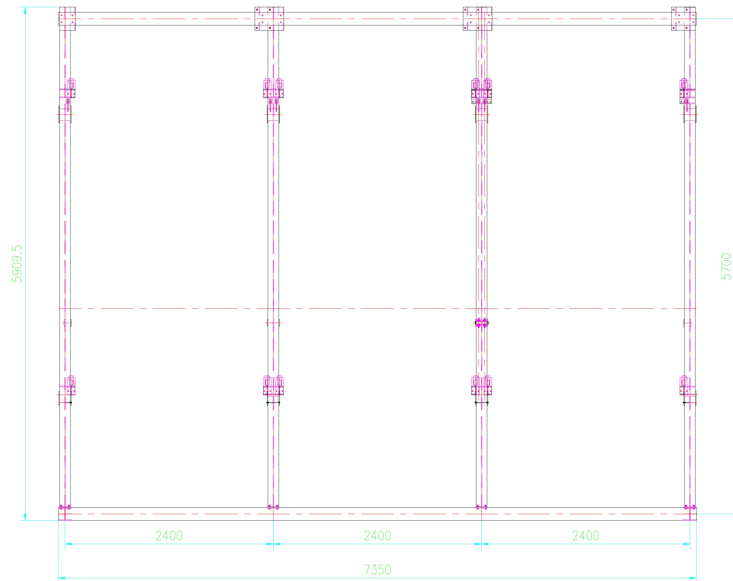
俯视图
