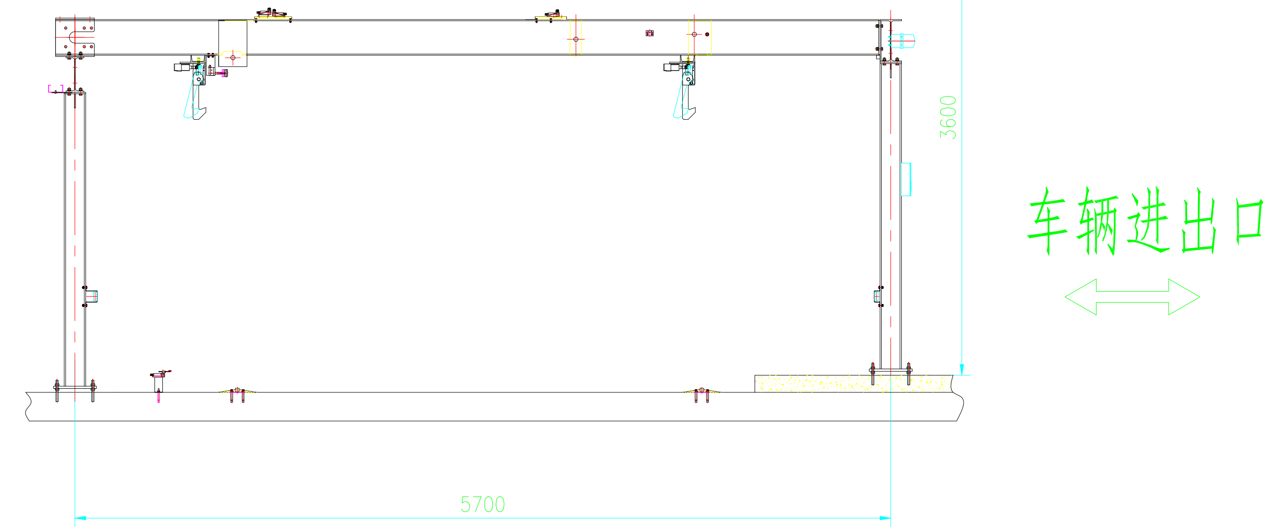
侧视图
