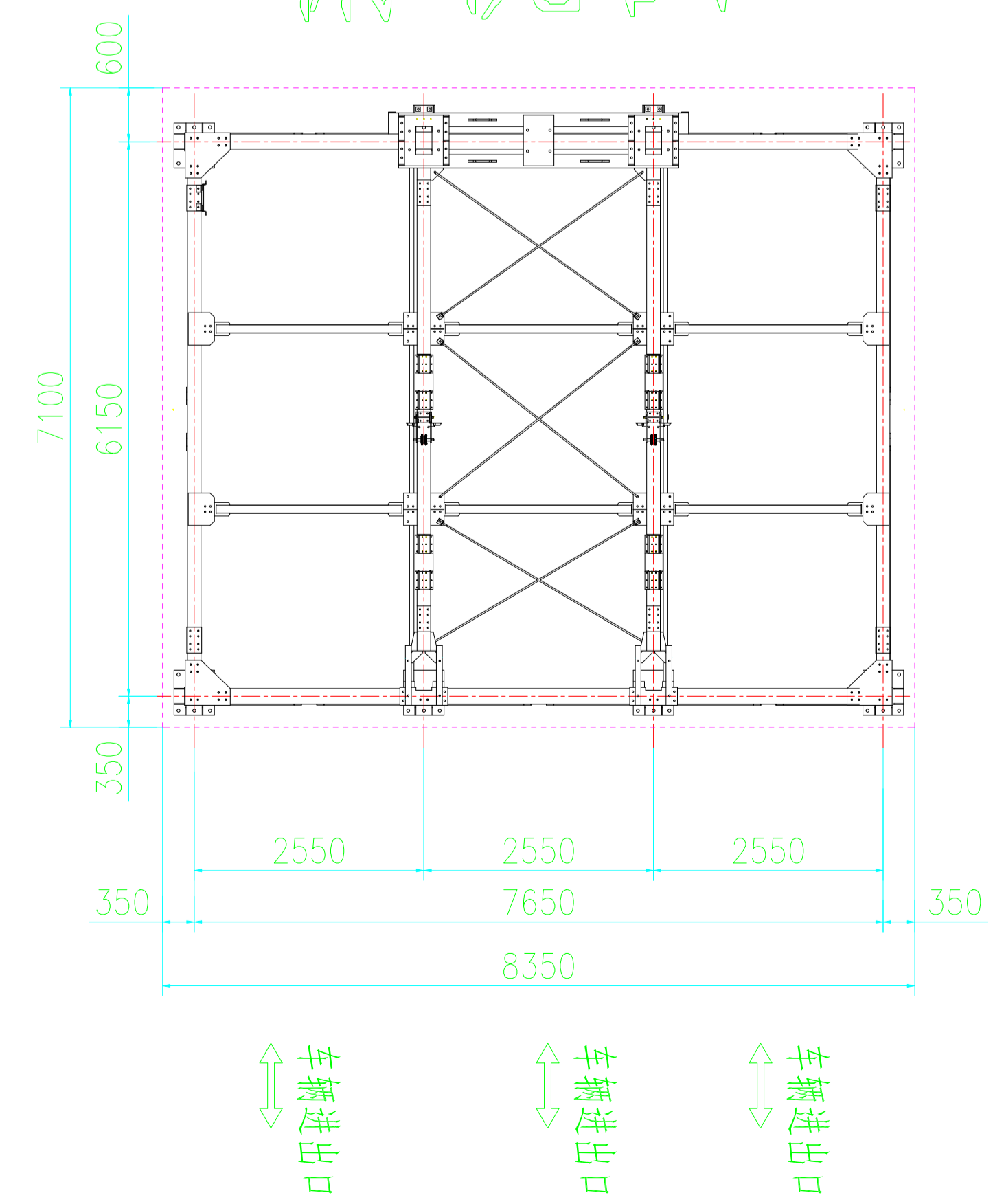
俯视图
