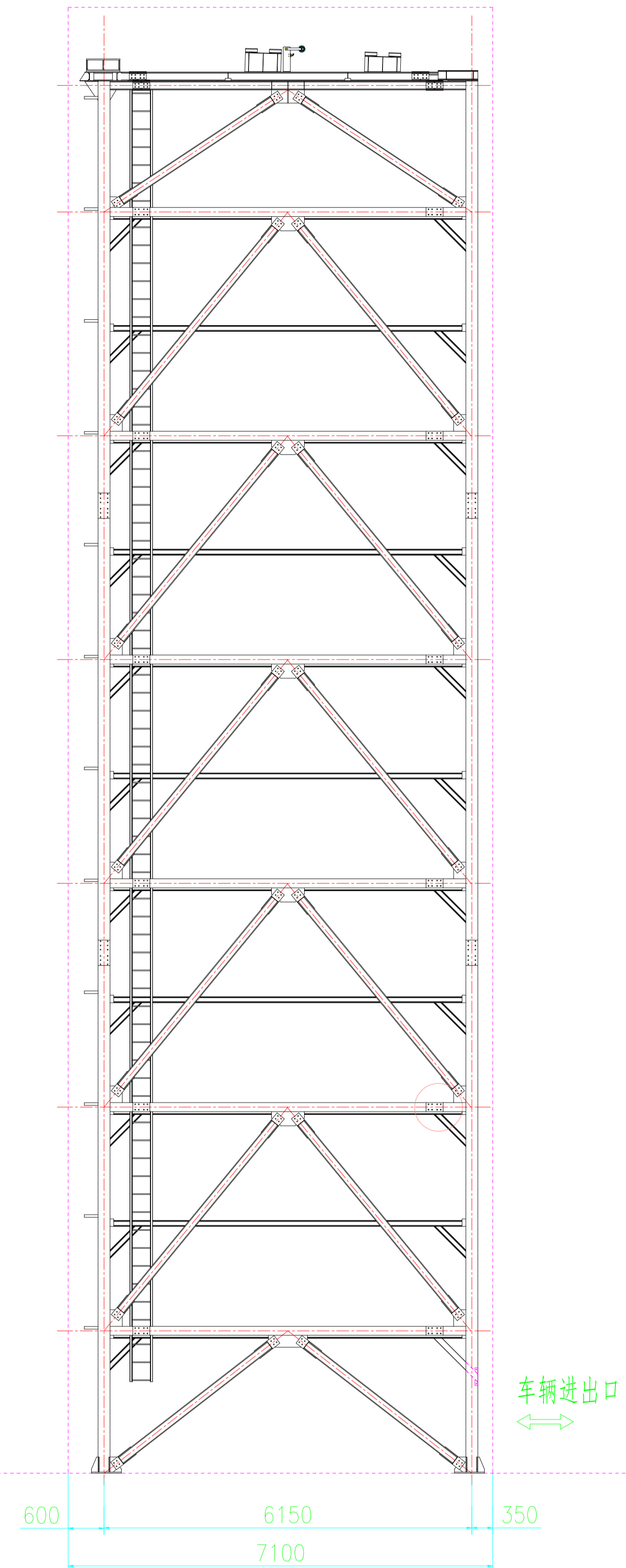
侧视图
